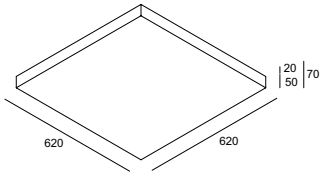
JETI PLANO L 424 271 52 424 G5 / 220-240V / 0 | 50-60Hz / 1 x 4~EVG 4 x T16 24W ◊ CE 5,9 IP20 0,1
