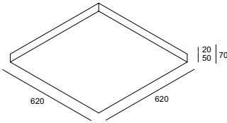
JETI PLANO L 160 271 52 160 2GX13 / 220-240V / 50-60Hz / 1 x 1~EVG 1 x T16-R 60W ◊ CE 5,4 IP20 0,1
